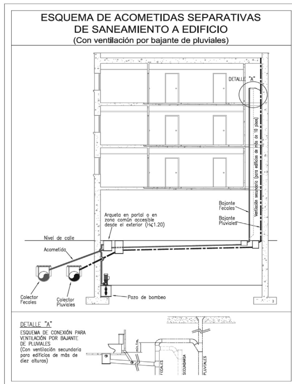
Esquema de acometidas separativas de saneamiento a edificio
