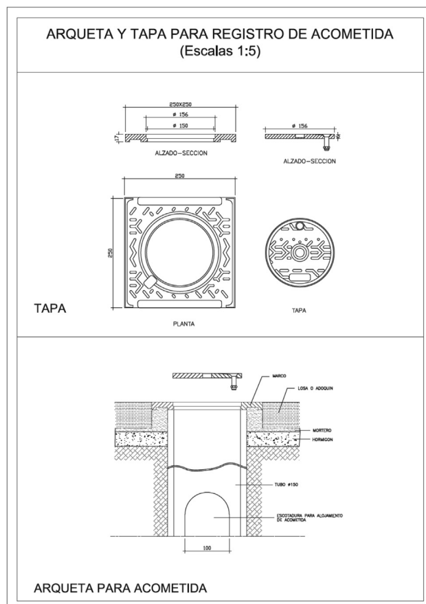
Arqueta y tapa para registro de acometida (Escala 1:5)
