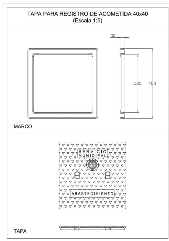
Tapa para registro de acometida 40 x 40
