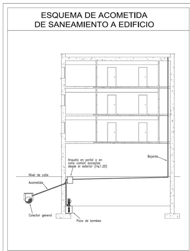
Esquema de acometidas separativas de saneamiento a edificio
