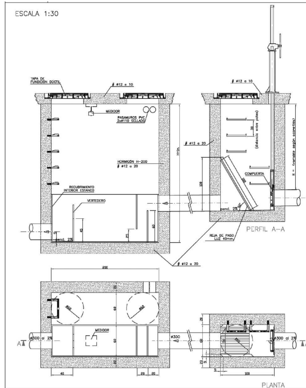
Arqueta de toma de muestras Tipo B con bombeo
