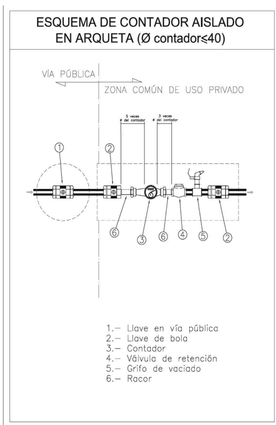
Arqueta tipo para contador (Dimensiones)
