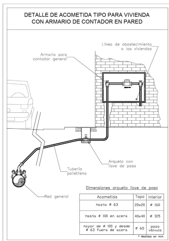
Arqueta tipo para contador (Dimensiones)
